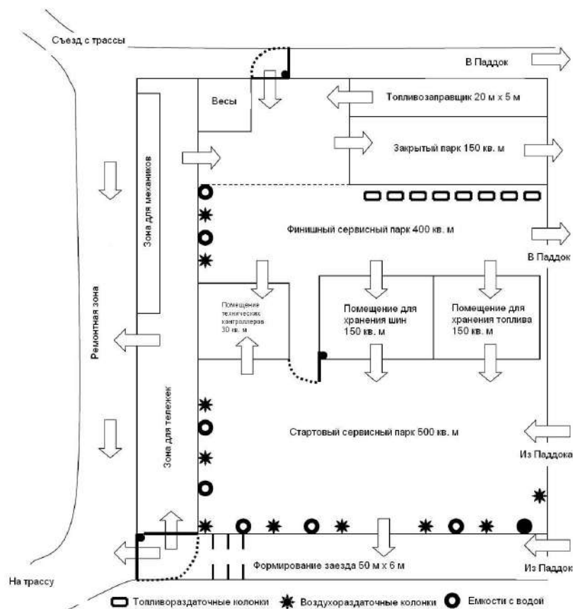
Рисунок 8 - Рекомендуемая планировка сервисного и закрытого парка
