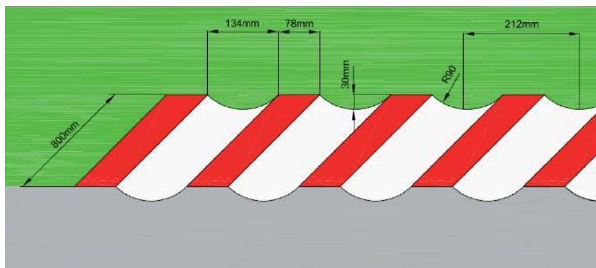
Рисунок 3 – Внешний поребрик для международных соревнований
