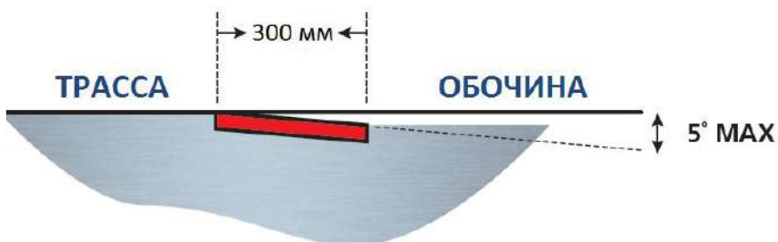
Рисунок 4 – Внешний поребрик, допустимый для трасс категории лицензии «С», «D» и «E»
