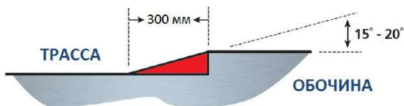
Рисунок 2 – Внутренний поребрик, допустимый для трасс категории лицензии «С», «D» и «E»
