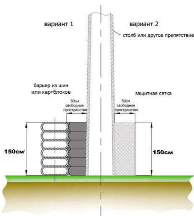
Рисунок 7 – Пример ограждения опасных структур, расположенных перед первой линией защиты
