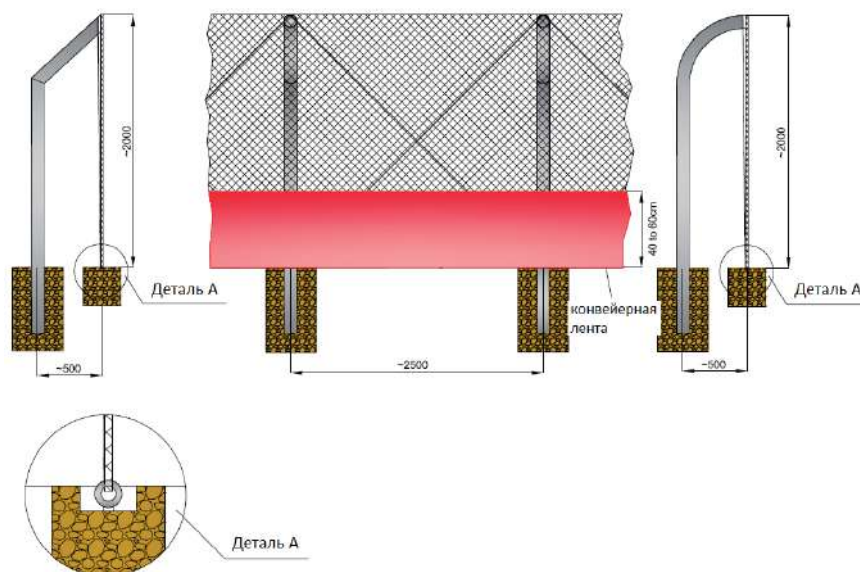
Рисунок 6 – Сетчатое ограждение
