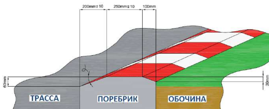
Рисунок 1 – Внутренний поребрик для международных соревнований
