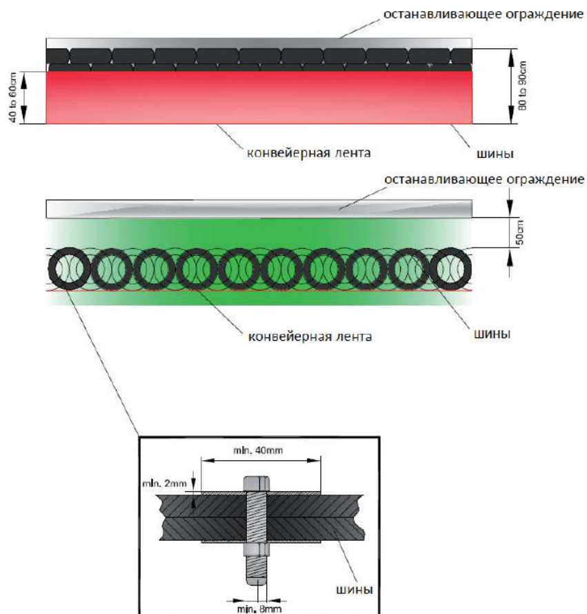
Рисунок 5 – Шинное ограждение
